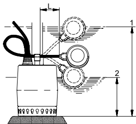
Käivitus- ja seiskamistasemed, UNILIFT KP-A
