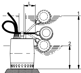
Niveluri de pornire și oprire, UNILIFT KP-A
