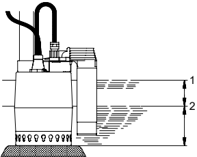
Indítási és leállítási szintek, UNILIFT KP-AV
