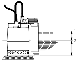
Ein- und Ausschaltniveau, UNILIFT KP-AV
