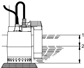
Razine pokretanja i zaustavljanja, UNILIFT KP-AV
