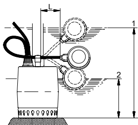
Старт и стоп нивоа, UNILIFT KP-A
