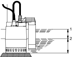
UNILIFT KP-AV 启动和停止液位
