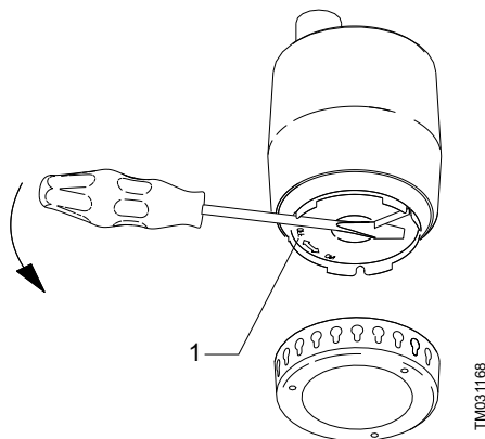
如何拆除泵壳
