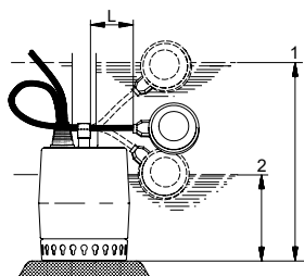
Στάθμες εκκίνησης και παύσης, UNILIFT KP-A
