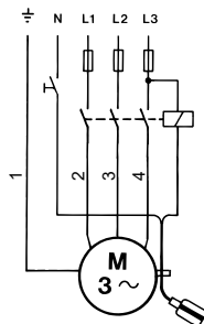
Savienojumu shēma
