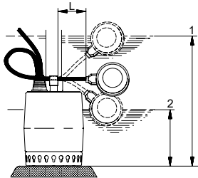
Nivoji vklopa in izklopa, UNILIFT KP-A
