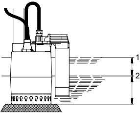
Нива за стартиране и спиране, UNILIFT KP-AV
