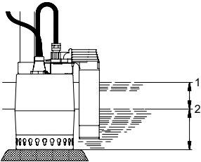
Livelli di avviamento e arresto, UNILIFT KP-AV
